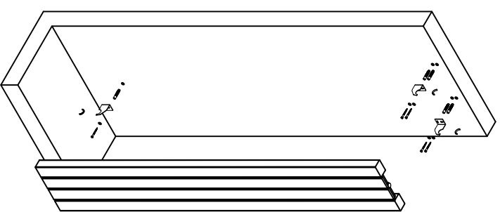
L=298 mm
